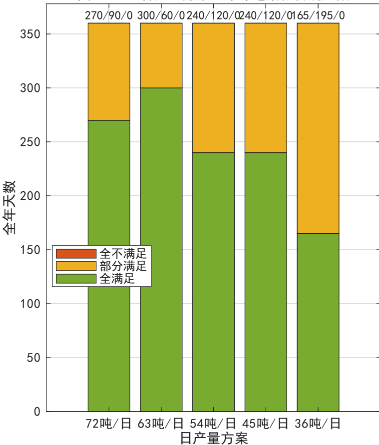
图 4(a) 各产量方案全年绿电指标合规天数
